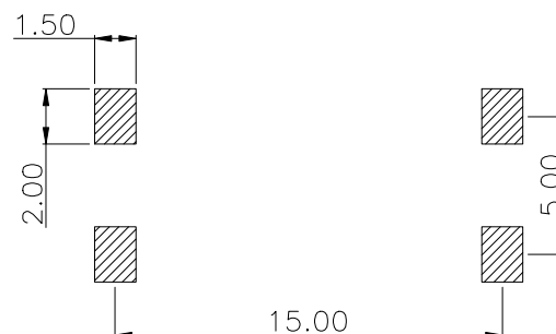
PCB.焊接图
