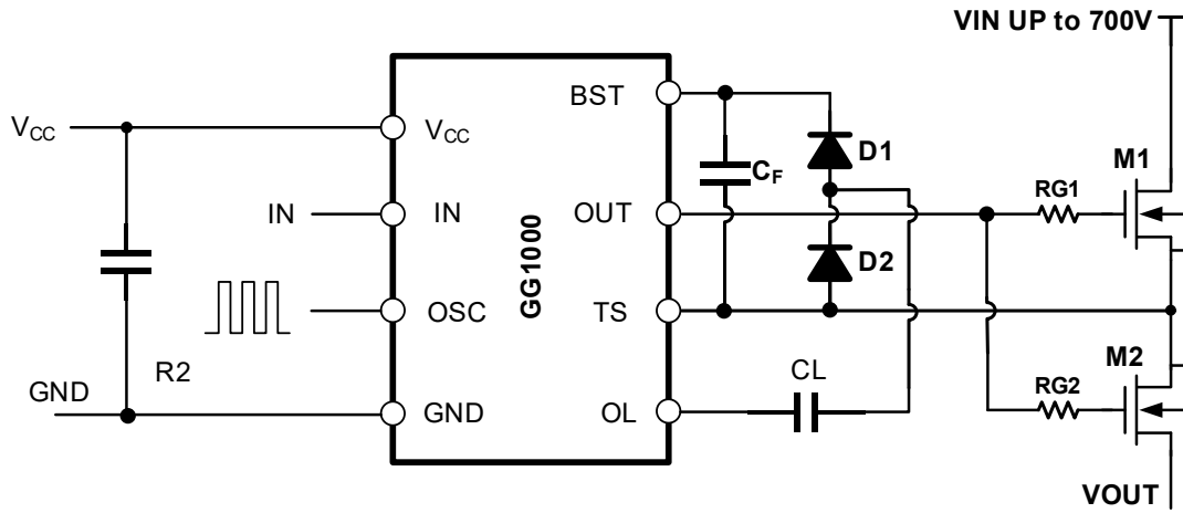
图 10-3 典型应用电路图 2
