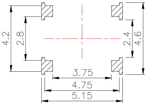
PCB.焊接图
