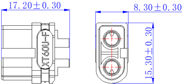
堆叠尺寸
