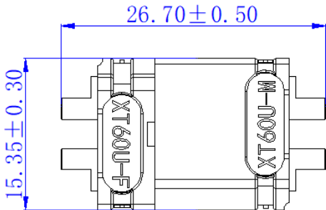
互配尺寸
