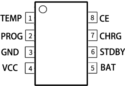
ESOP-8
