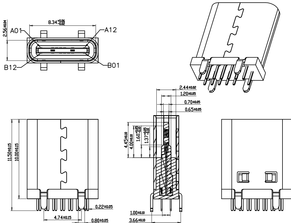
截面 1-1
