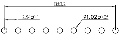
P.C.B LAYOUT
