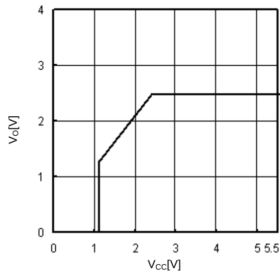
Fig.15 V_{CC}-V_O ( I_O=0mA )
