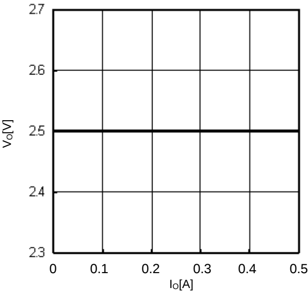
Fig.13 I_O - V_O
