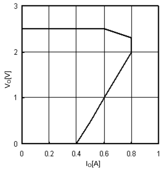
Fig.17 OCP
