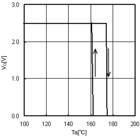
Fig.16 TSD ( I_O=0mA )
