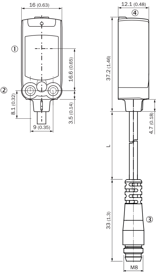
尺寸图 (尺寸单位: mm)
