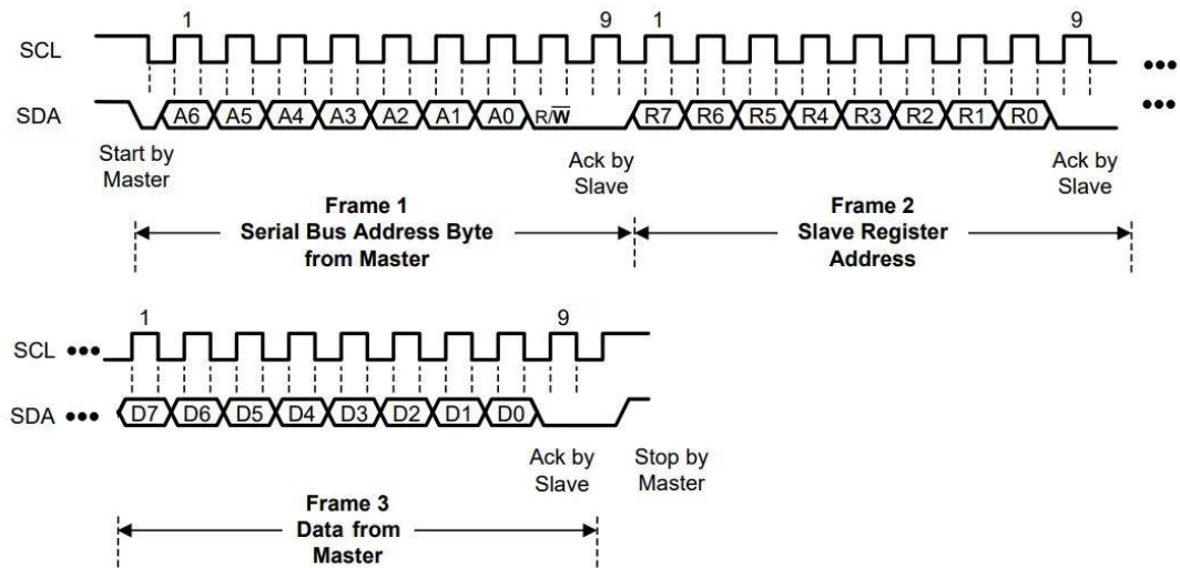
图 7.2-3 I2C 写时序
