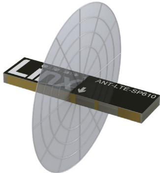
YZ-Plane Gain
