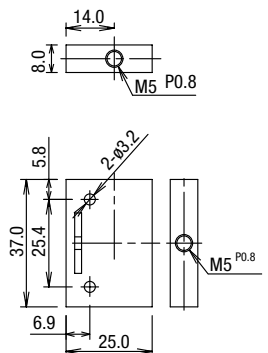
SA9Z-A02
