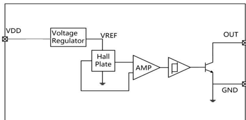
AH421 功能框图
