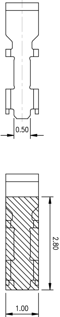
焊盘尺寸
