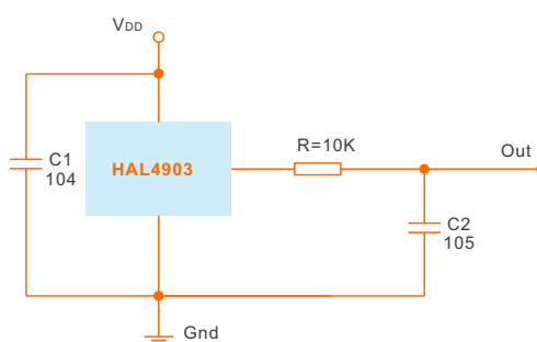
低噪声应用
