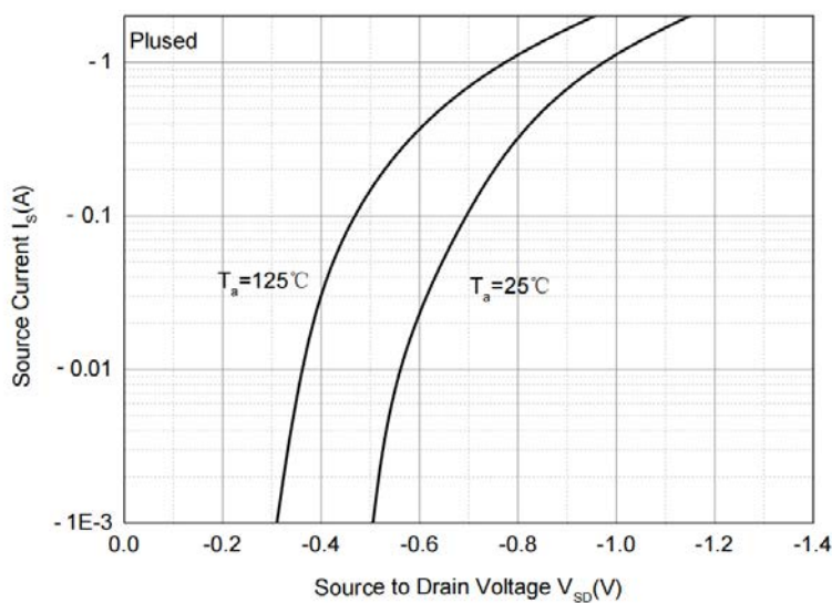
I_S - V_{SD}
