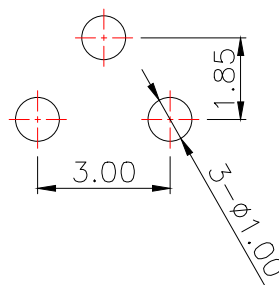
PCB.焊接图
