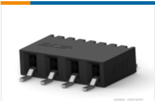
TE Part #284513-4 4 POS TERMI-BLOK HDR 900 POL.
