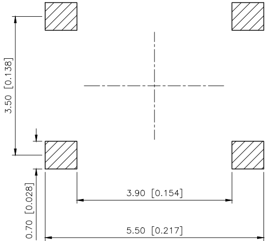
P.C.B LAYOUT
