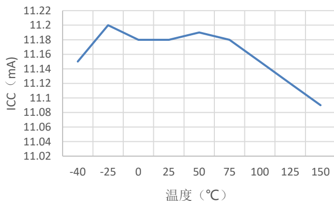
平均电流随温度变化
