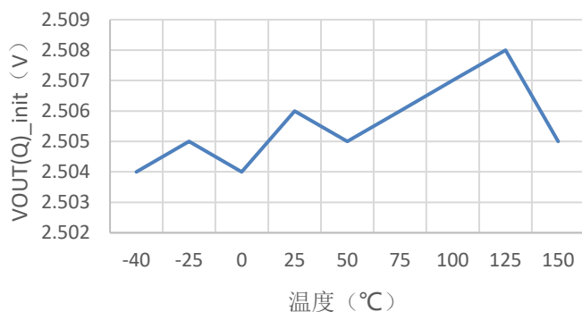
0Gauss磁场，静态输出输出随温度变化
