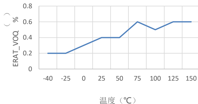
静态输出误差随温度变化
