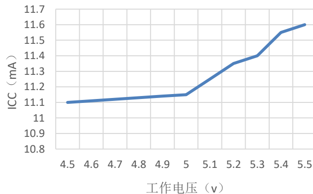
平均电流随工作电压变化
