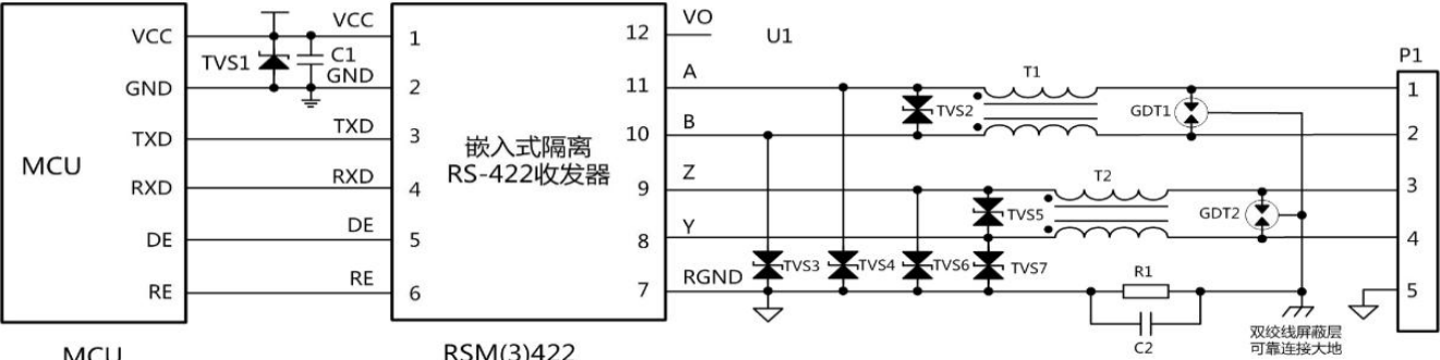
图 2. EMC 推荐电路
