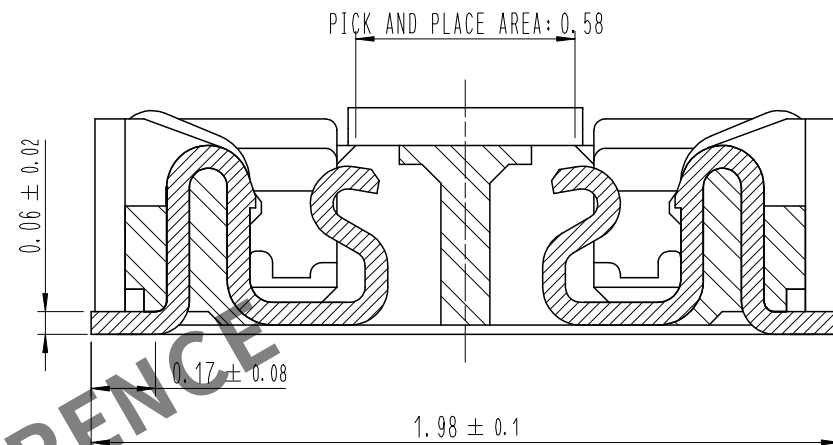
A-A (50:1)
