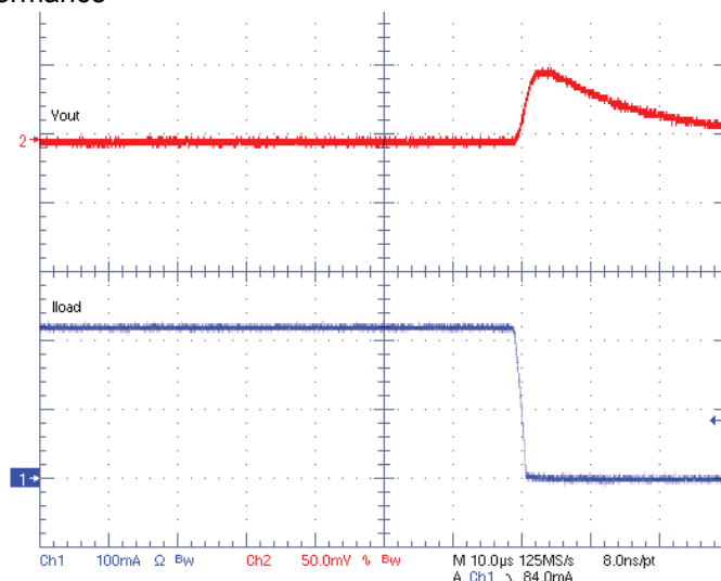
LDO3 - VIN = 5.5V - VDD3 = 3.3V Load Step 200 To 0mA / 1µs
