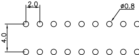
P.C.B LAYOUT
