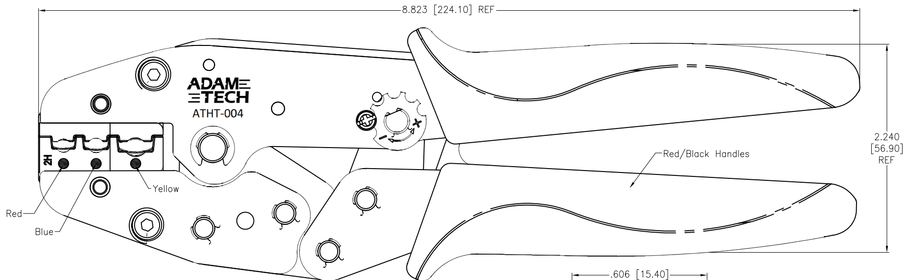
CRIMP DIE
