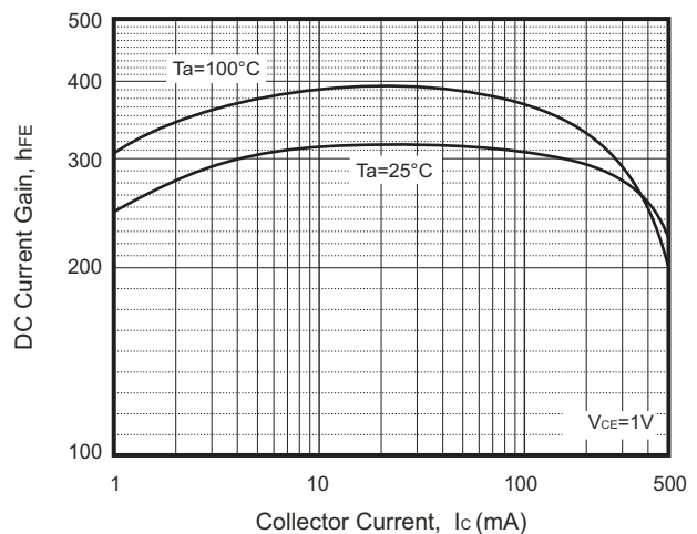
Fig.2 - h_{FE} - I_C
