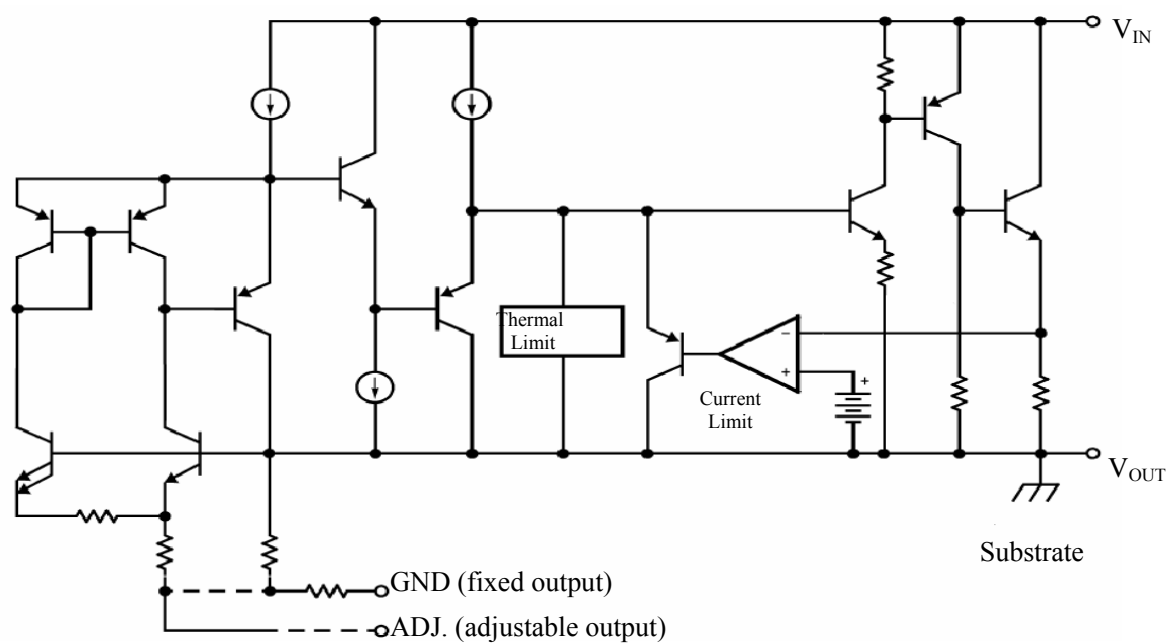
功能图
