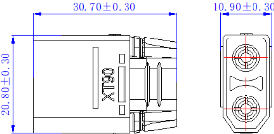
互配尺寸
