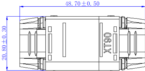
带后盖互配尺寸
