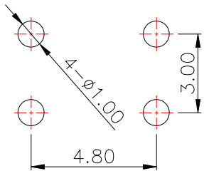
PCB.焊接图
