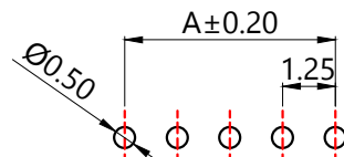
适用线路板 (PCB LAYOUT)
