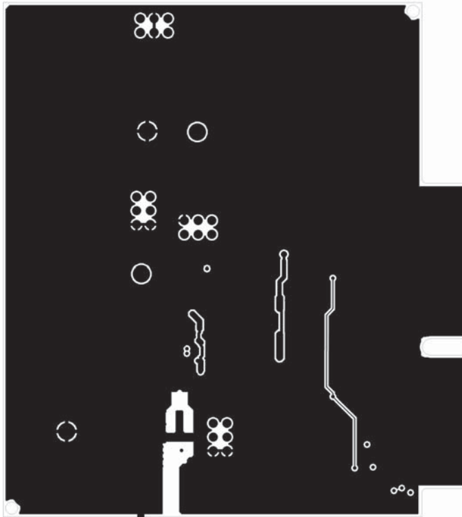
Layer 5 GND
