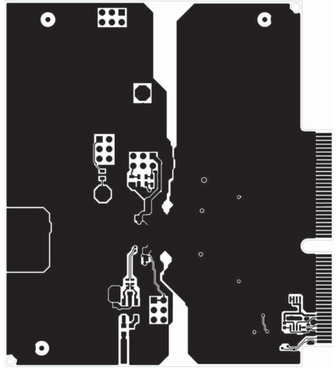
Layer 6 Bottom Side
