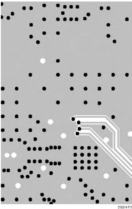
Inner Layer 3
