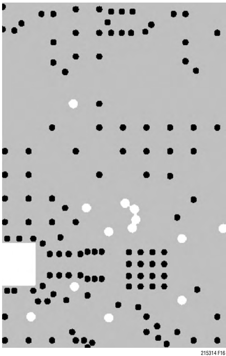
Inner Layer 2
