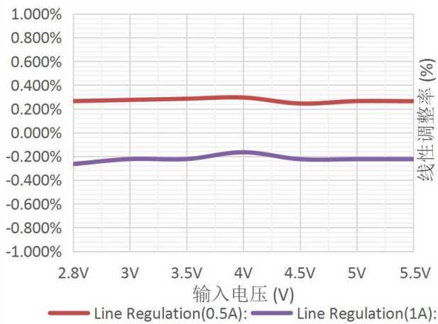
线性调整率
