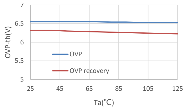
OVP vs T_a
