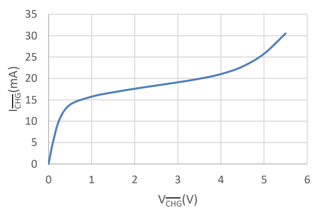
I_{\text{CHG}} \text{ vs } V_{\text{CHG}}
