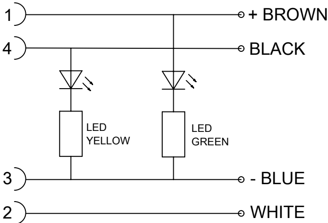
PNP WIRING
