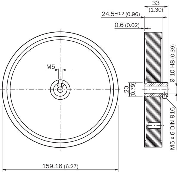
尺寸图 (尺寸单位: mm)
