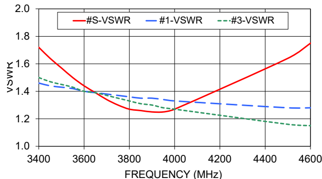
WP4S+ VSWR
