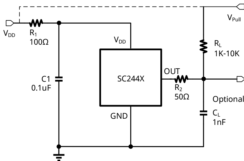
图 6：典型应用线路图
