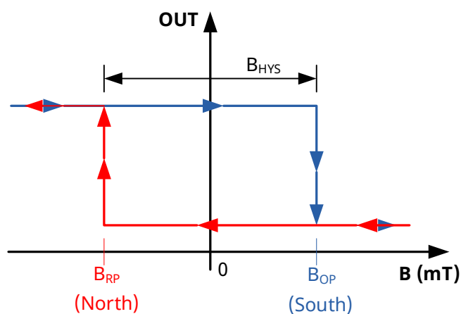
图 5: UA 封装传输曲线图
