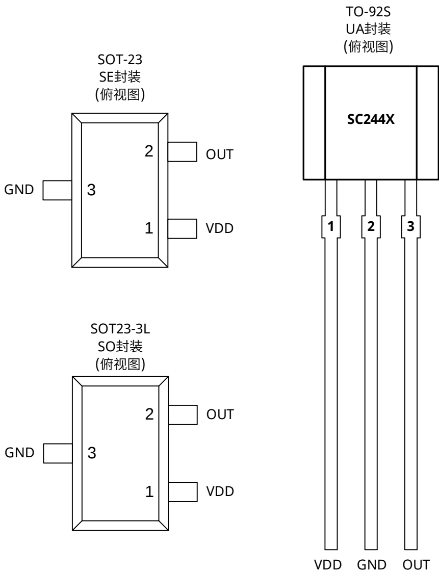
图 2：引脚定义图
