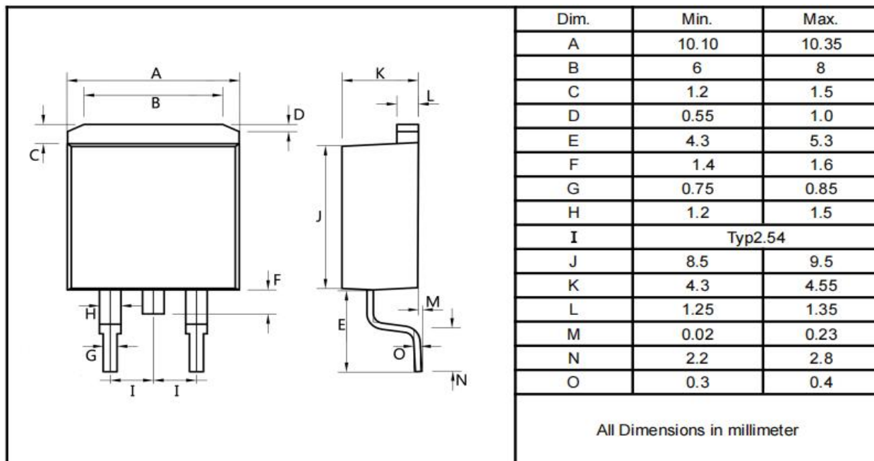
TO-263
