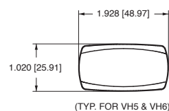
(TYP. FOR VH5 & VH6)
