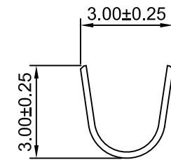
SEC:A-A
