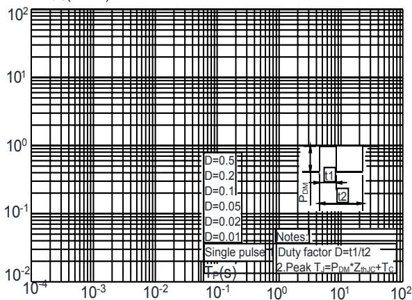
Z_{th_{J-C}}(^{\circ}C/W)
