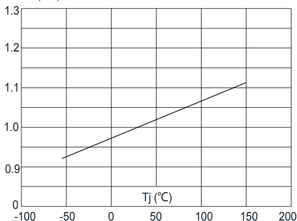
V_{BR(DSS)}
