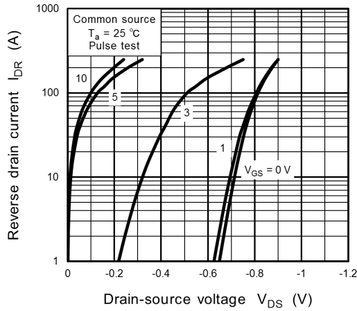
Fig. 9.7 I_{DR} - V_{DS}
