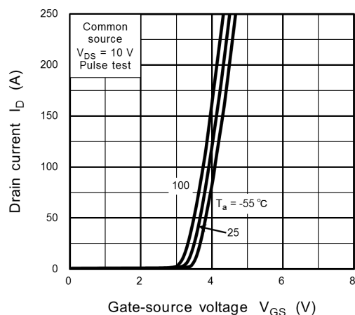
Fig. 9.3 I_D - V_{GS}
