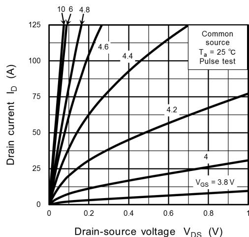
Fig. 9.1 I_D - V_{DS}
