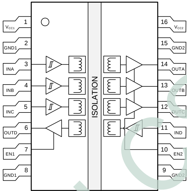
引脚功能
