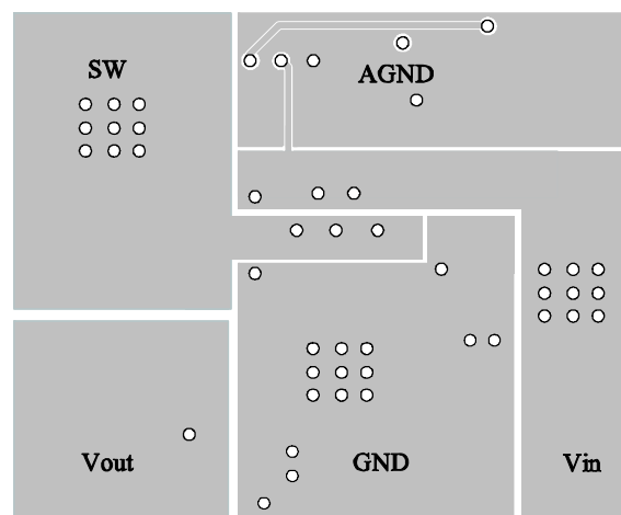
Inner2 Layer
