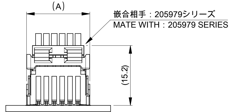
△ 4 ISLタイプ嵌合図 MATED CONNECTOR OF ISL TYPE
