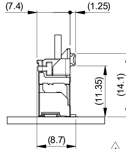
△ 4 ISLタイプ嵌合図 MATED CONNECTOR OF ISL TYPE
