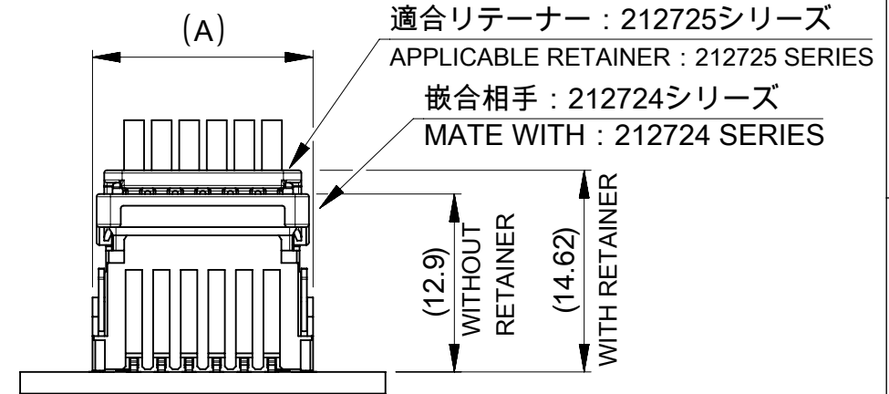
△ 4 TPAタイプ嵌合図 MATED CONNECTOR OF TPA TYPE
