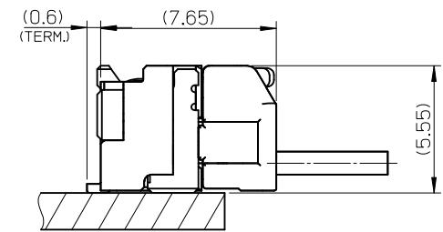
嵌合図
