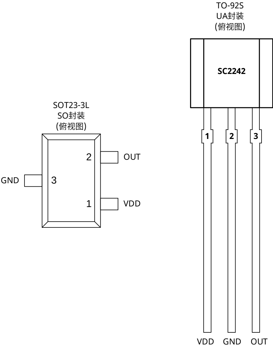
图 2 引脚描述
