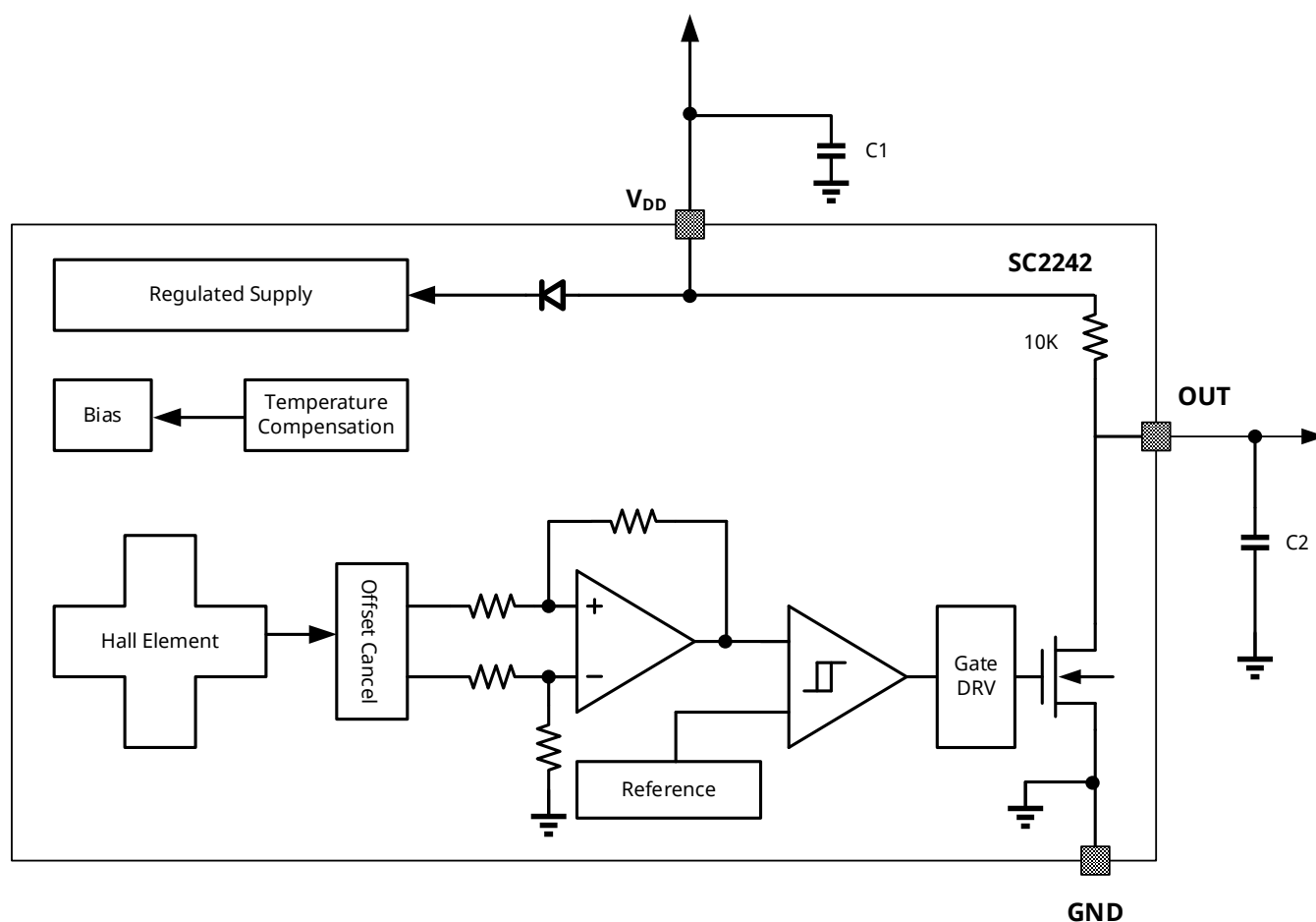
图 3 功能框图
