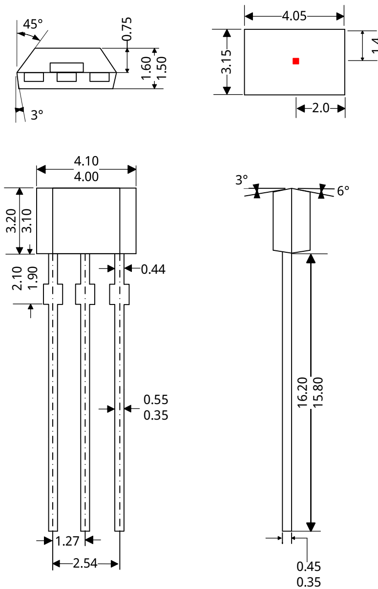
3-脚 S3 封装
