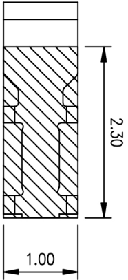
焊盘尺寸
