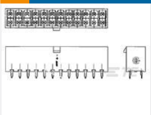
TE Part #1586768-4 4P VERT HDR VAL-U-LOK GW
